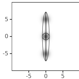
Phase-Space
