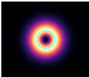
QHO n=1
