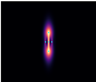
2-cat
