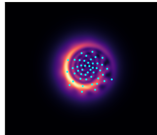
Kerr
