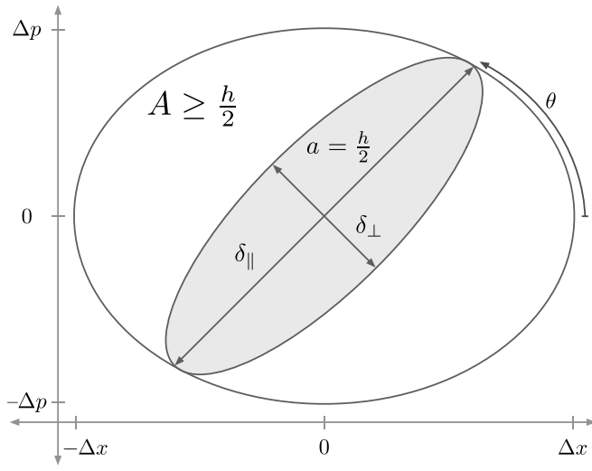
FIG. 1. de Gosson cells
