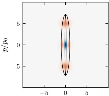
Wigner Phase-Space
