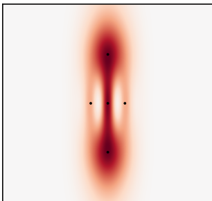
2-cat
