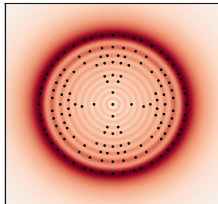
Kerr
