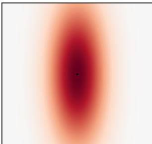
2-cat
