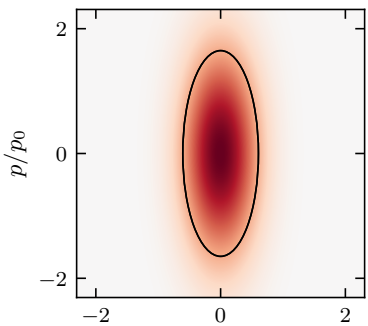
Wigner Phase-Space
