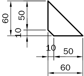
K6 耳板三角筋板 t8 ×4 Q355B 0.11kg/件 直角处 10×10 清角
