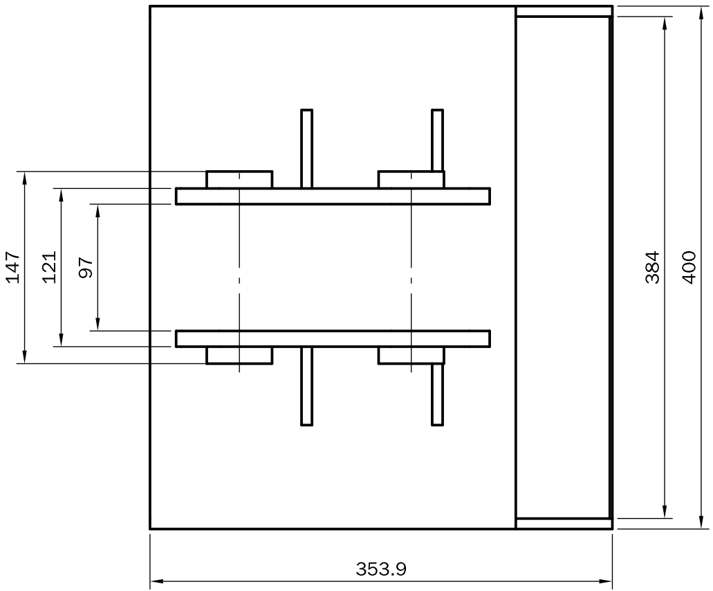
K5 斗耳板 t12 ×2 Q355B 2.08kg/件
