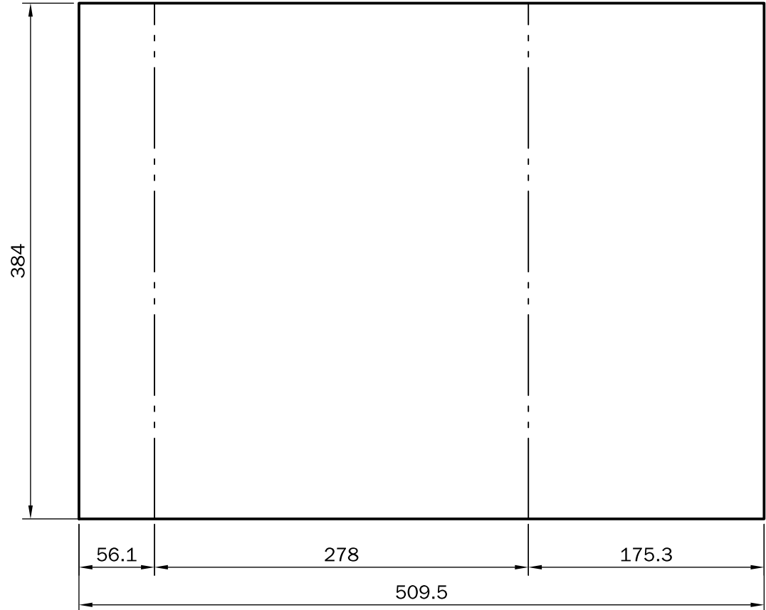
K4 底弧板 t6 ×1 Q355B 9.21kg/件 两点划线之间卷弧 : 中性层 R177 / 内 R174 (90°) 线外两段保持平直
