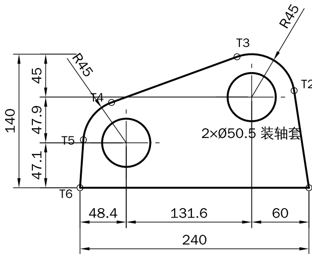
K5 斗耳板 t12 ×2 Q355B 2.08kg/件
