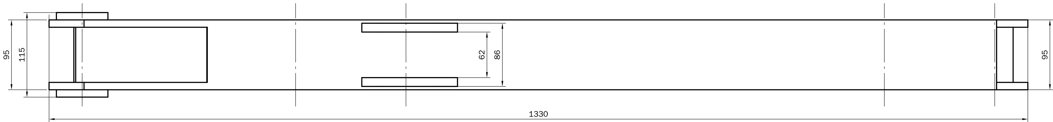
俯视图
