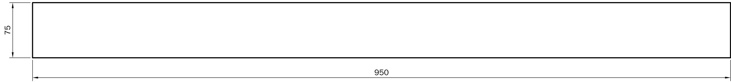
A2 臂底板 t12 ×1 Q355B 6.71kg/件
