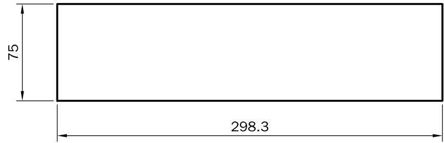
A4 臂后板 t10 ×1 Q355B 1.76kg/件
