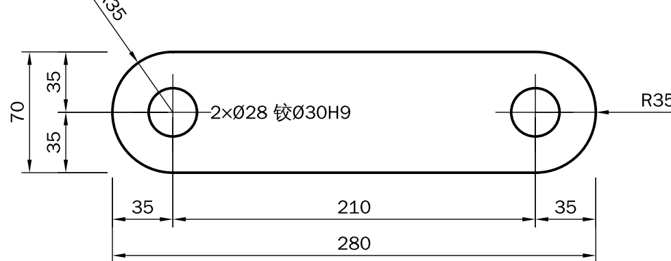
L2 铲斗连杆 t10 ×2 Q355B 1.36kg/件
