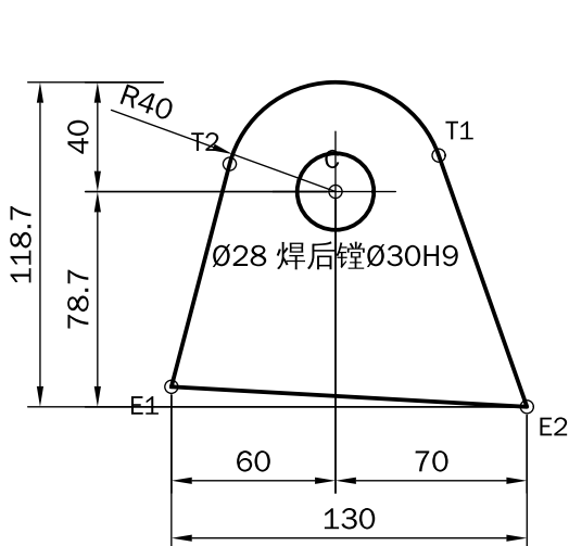
A5 斗缸耳板 t12 ×2 Q355B 0.93kg/件
