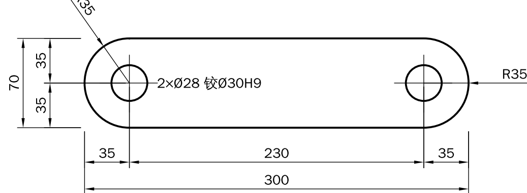
L1 斗杆连杆 t10 ×2 Q355B 1.47kg/件
