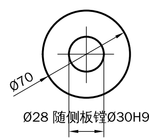
A6 B处加强环 t10 ×2 Q355B 0.25kg/件
