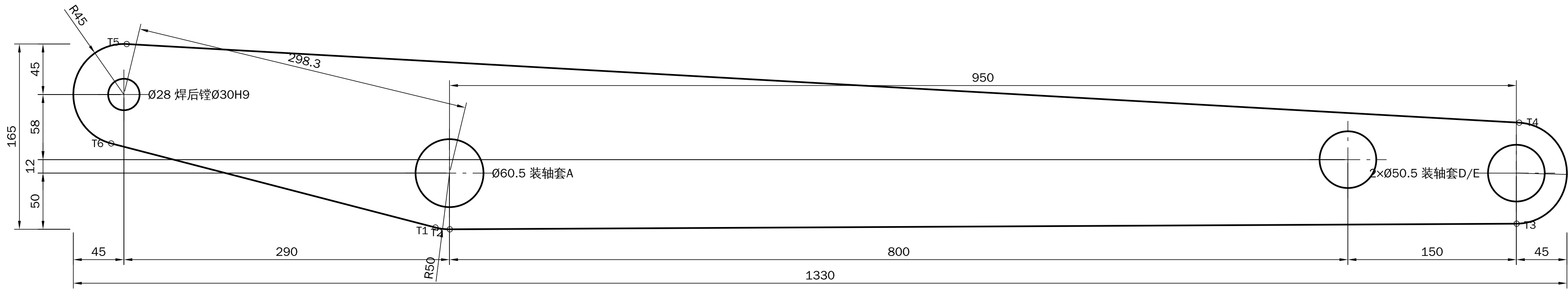
A1 臂侧板 t10 ×2 Q355B 11.57kg/件
