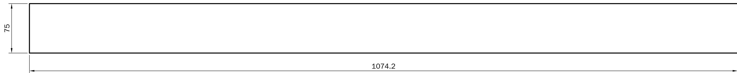
A6 B处加强环 t10 ×2 Q355B 0.25kg/件
