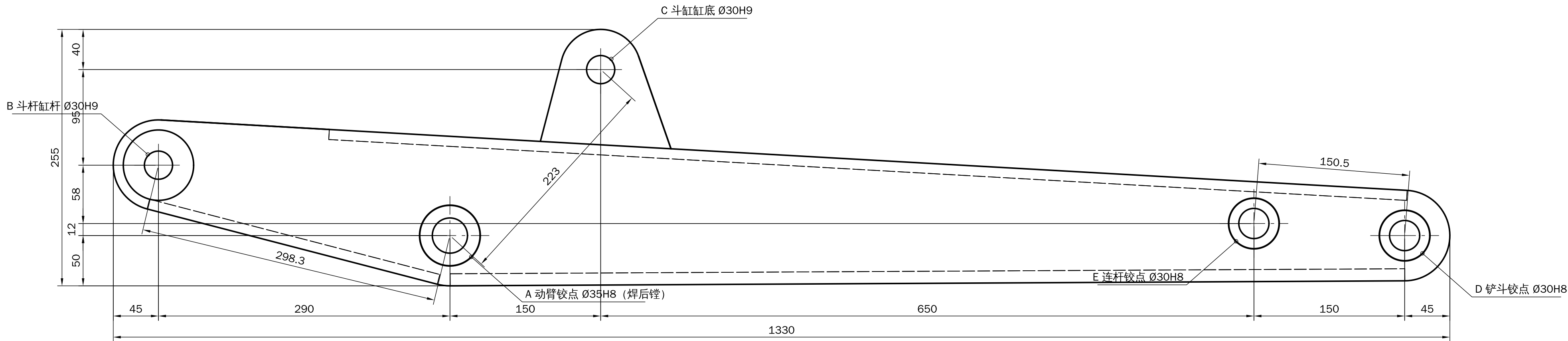
主视图
