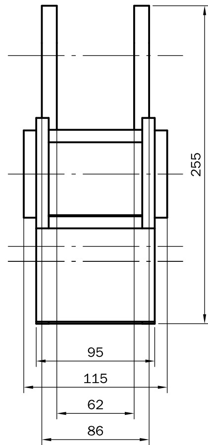
左视图
