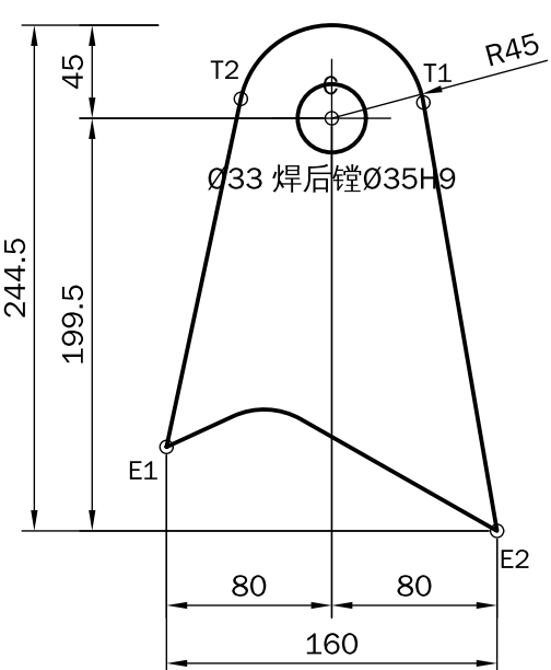
B5 臂缸耳板 t16 ×2 Q355B 2.78kg/件
