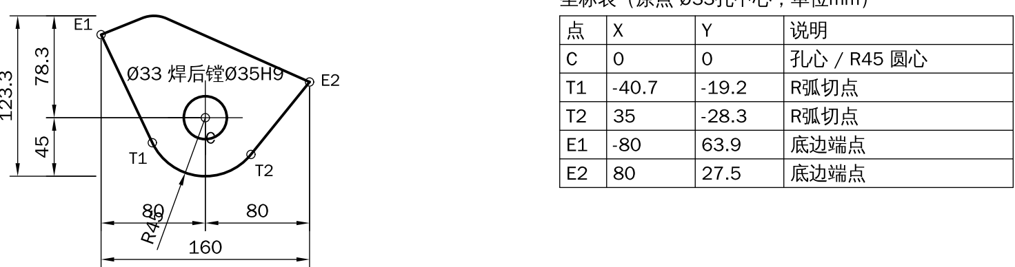
B4 动臂缸耳板 t16 ×2 Q355B 1.33kg/件
