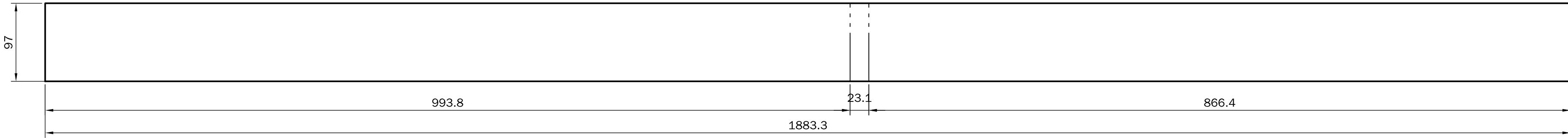
B3 动臂底板(腹板) t12 ×1 Q355B 17.21kg/件
