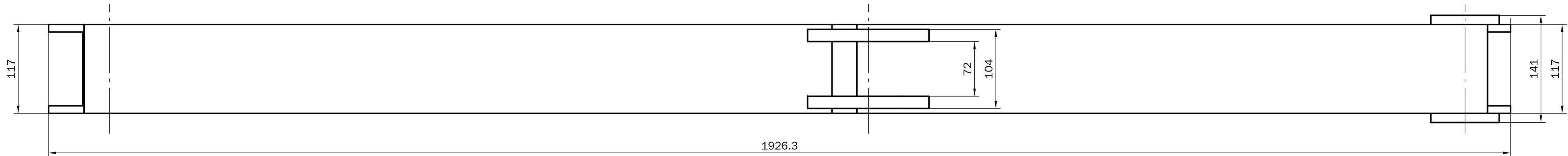
B1 动臂侧板 t10 ×2 Q355B 28.09kg/件
