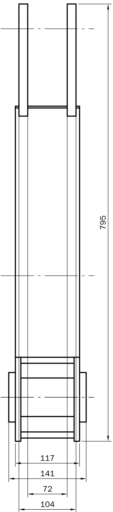
左视图
