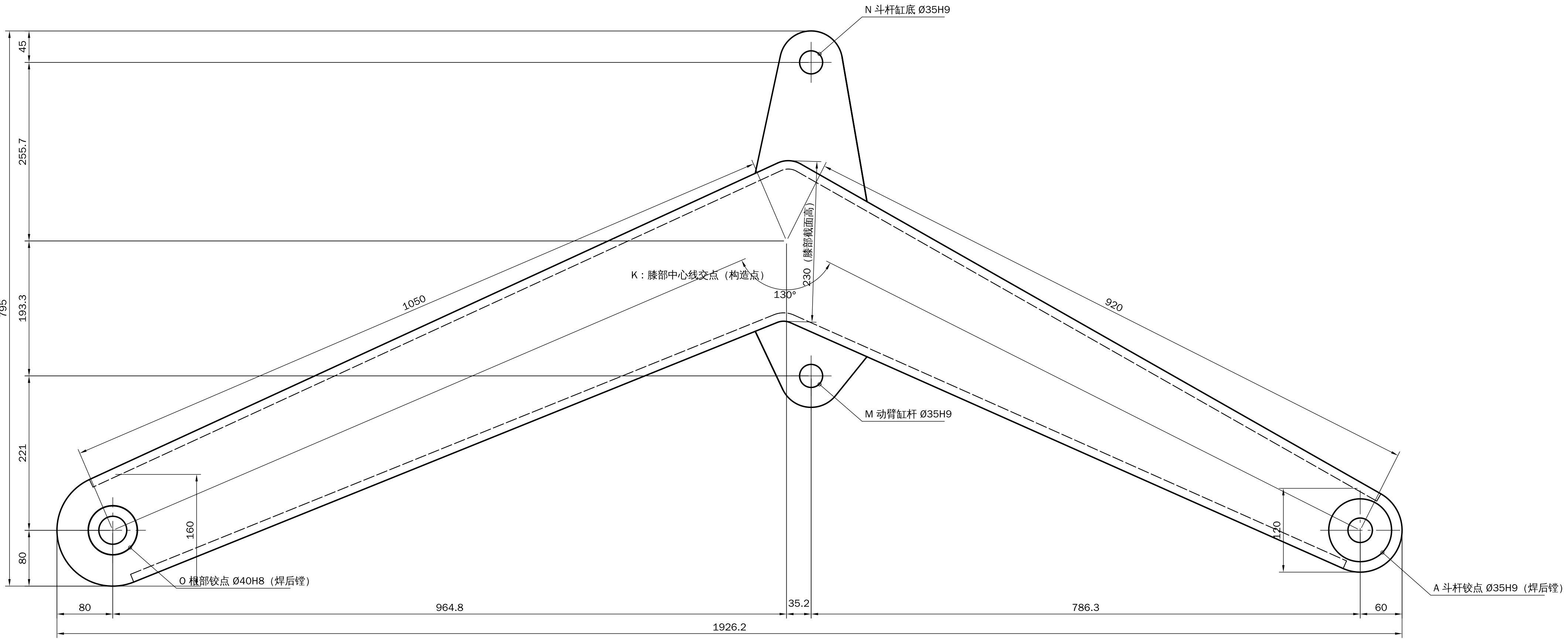
主视图
