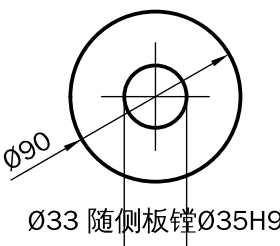
B6 臂销端环板 t12 ×2 Q355B 0.52kg/件
