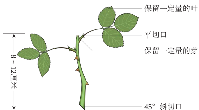
月季花枝条示意图
