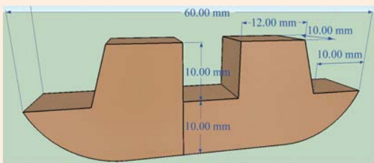
图 2.27 拱的参考尺寸
