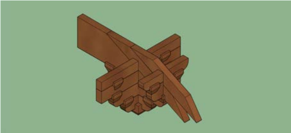
图 2.15 斗拱模型轴测图
