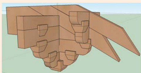
图 2.31 斗拱模型整体效果图
