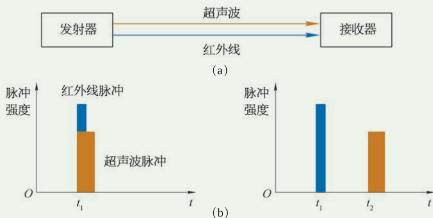
图 1-12 位移传感器测距离的原理示意图
