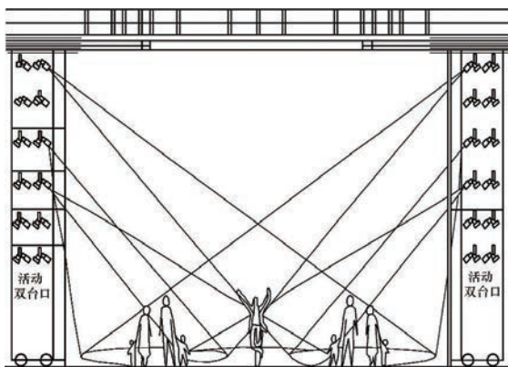
舞台上的灯光设备示意图
