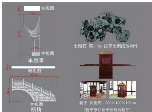
话剧《红楼梦》局部景物道具部分制作图：半扇亭、太湖石、断桥、轿子
