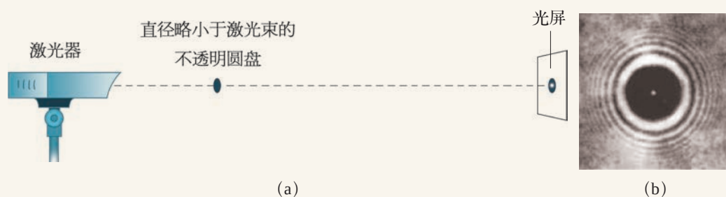
图 4-33 圆盘衍射
