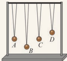
图 2-28 观察摆的受迫振动及共振装置
