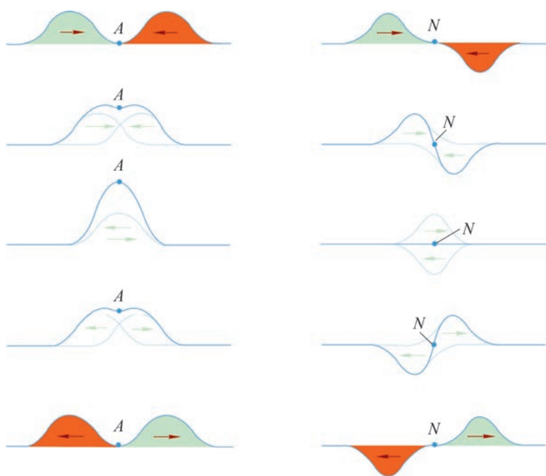
(a) 两个波峰在 A 点相遇
