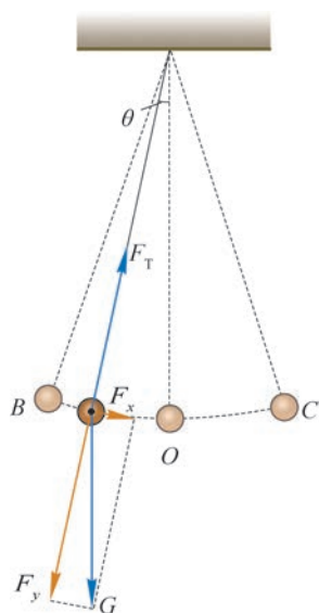
图 2-19 摆球的受力分析图
