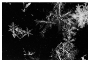
图 11-37 雪花
