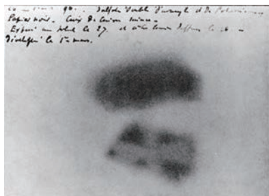
图 15-2 铀辐射照片
