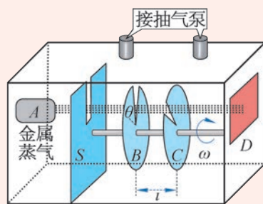
图 10-17 密勒和库士的实验装置示意图
