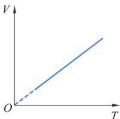
图 11-23 等压线
