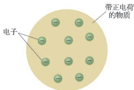
图 13-5 “枣糕模型”
