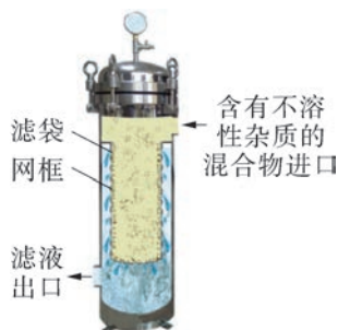
工业过滤器
