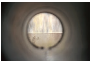
图 2.9 工业上氢气与氯气燃烧时火焰呈苍白色
