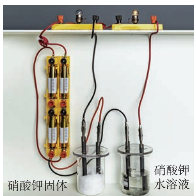
图 2.12 物质导电实验装置
