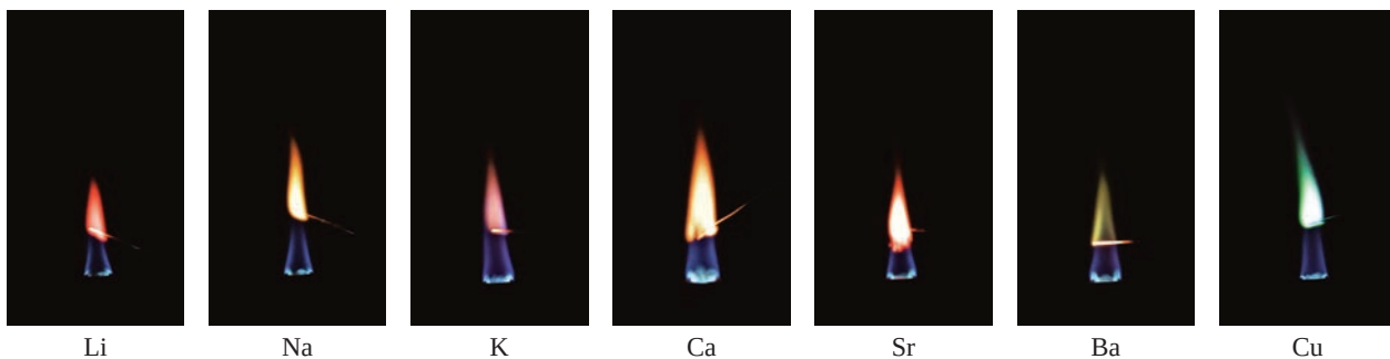
图 1.25 几种金属元素焰色试验的颜色
