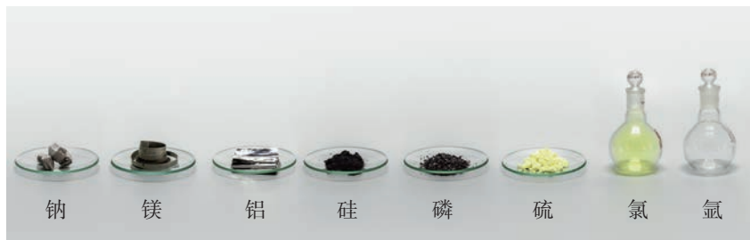
图 4.8 第 3 周期元素的单质
