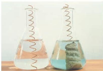
铜与硝酸银溶液的置换反应
