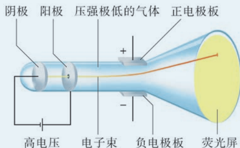
图 4.15 阴极射线管的简化结构图
