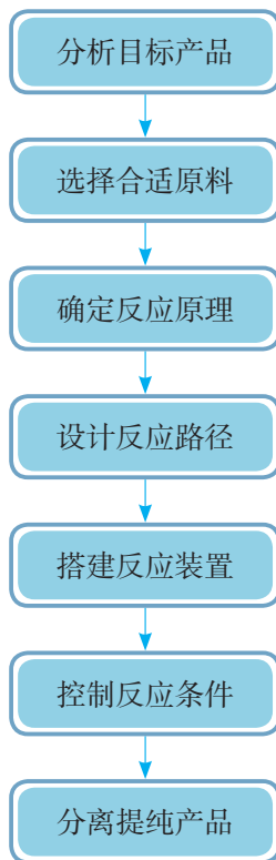
图 1.14 制备物质的一般流程
