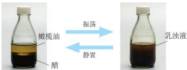
图 1.6 橄榄油和醋形成不太稳定的乳浊液
