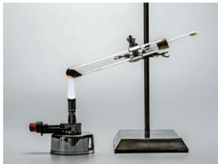
图 3.1 硫与铁的反应
