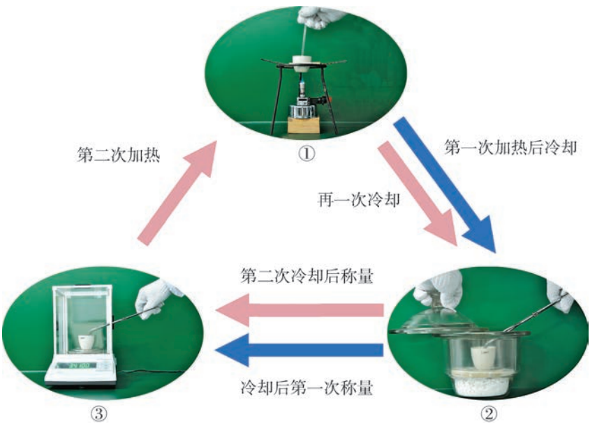
图 3.20 恒重操作
