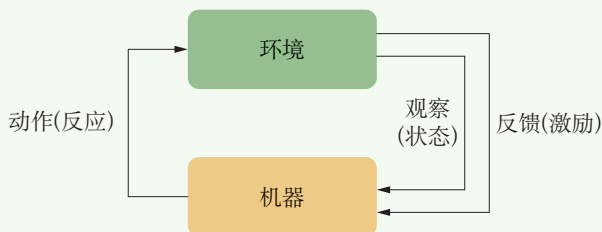
图 4.23 强化学习
