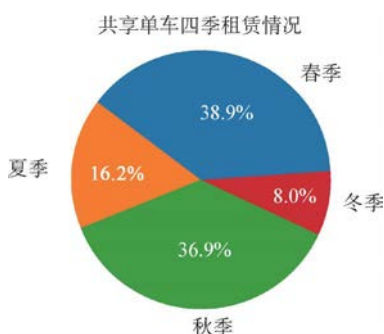
图 3.25 绘制饼图
