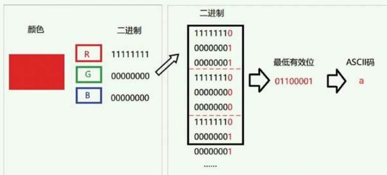
图 1.27 图像隐写术
