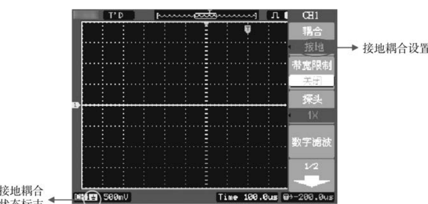
图 1-30 接地耦合设置下的波形显示
