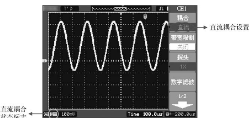
图 1-29 直流耦合设置下的波形显示
