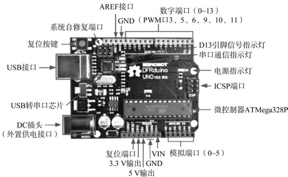
图 2-3 Arduino Uno
