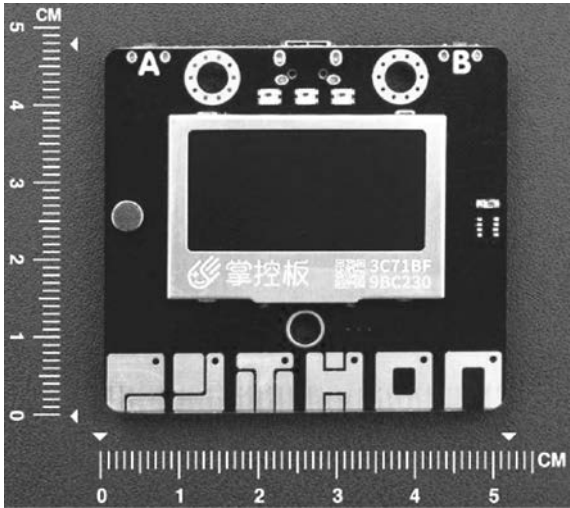
图 1-21 掌控板
