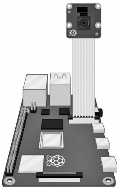
图 4-4 树莓派摄像头拍照
