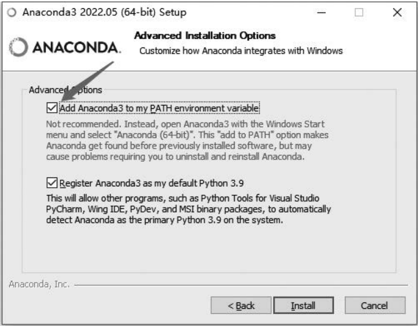
图 4-20 安装 Anaconda
