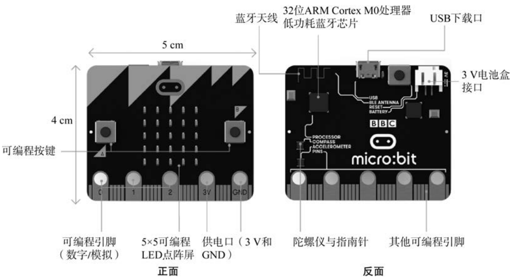
图 1-9 micro:bit 界面
