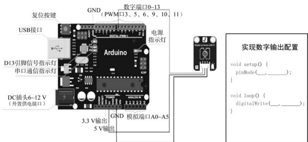
图 2-6 Arduino Uno 连接及输出配置
