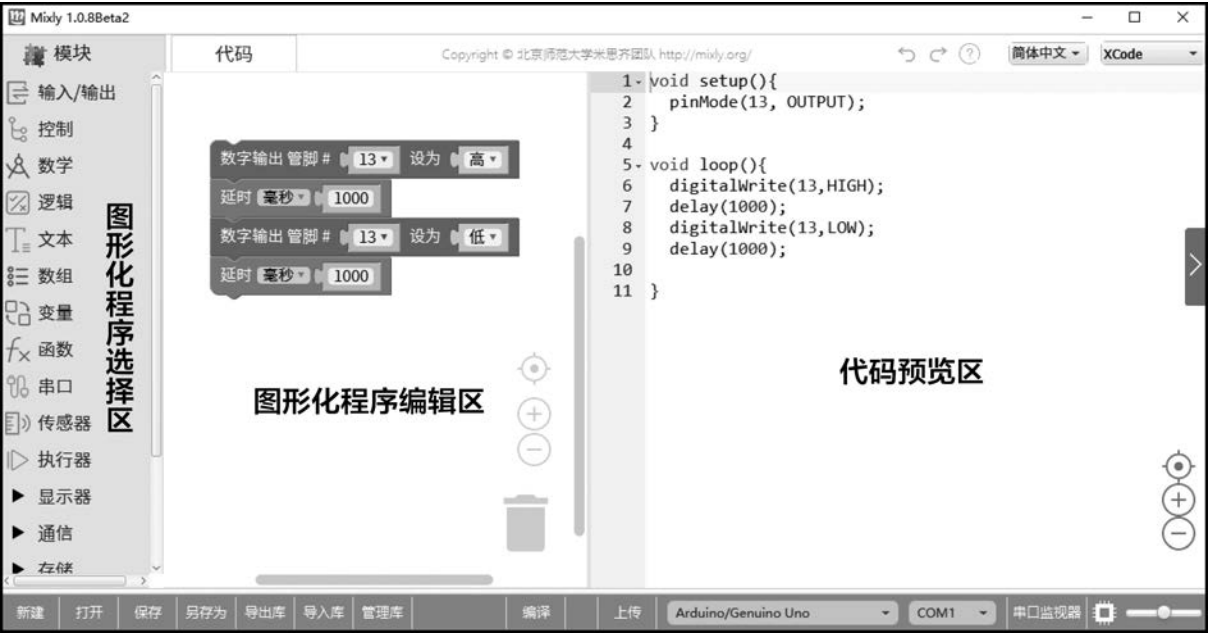
图 2-4 米思齐界面
