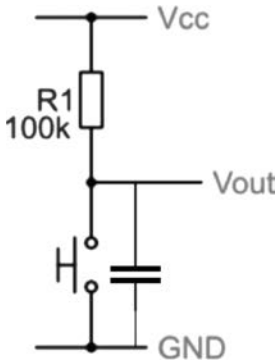
图 2-10 滤波电路线路
