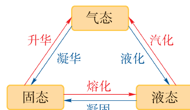
图 1.3 物质的三态变化
