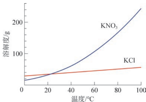
图 1.19 KCl 和 \text{KNO}_3 的溶解度曲线
