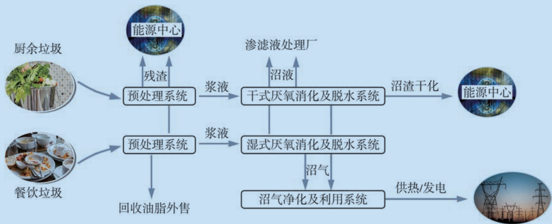
图 1-27 湿垃圾处理流程
