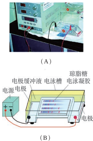
图 3-15 凝胶电泳示意图
