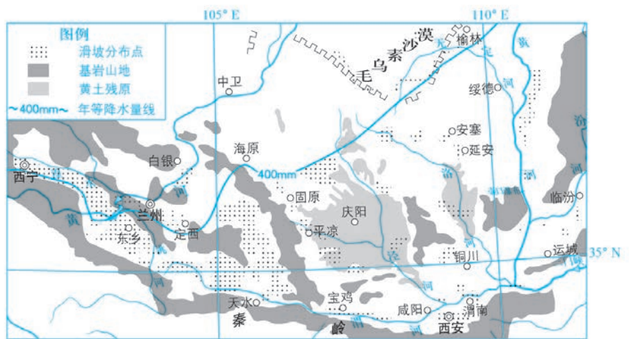
黄土高原滑坡分布图
