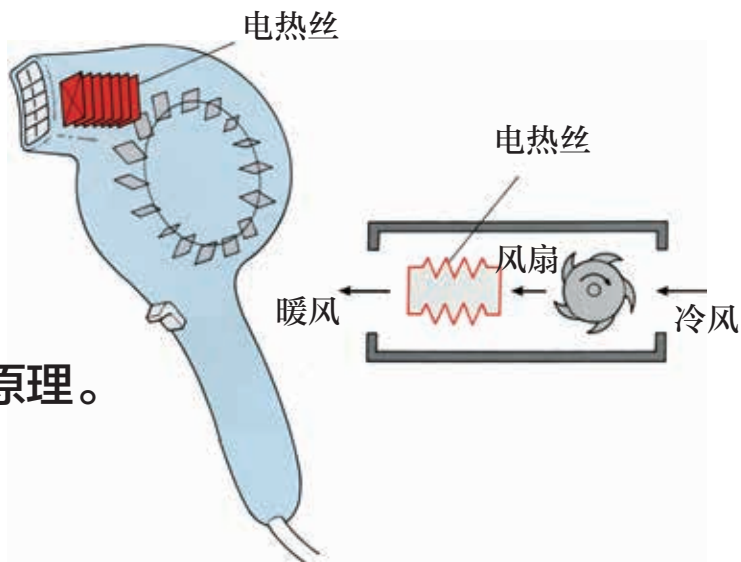
吹风机
