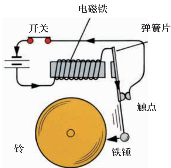
电铃示意图
