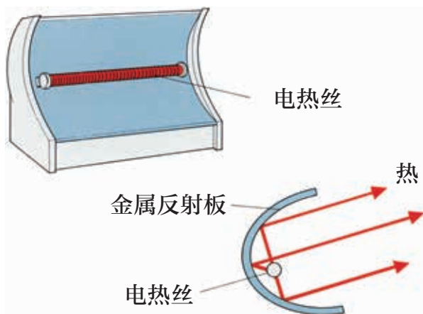
取暖器
