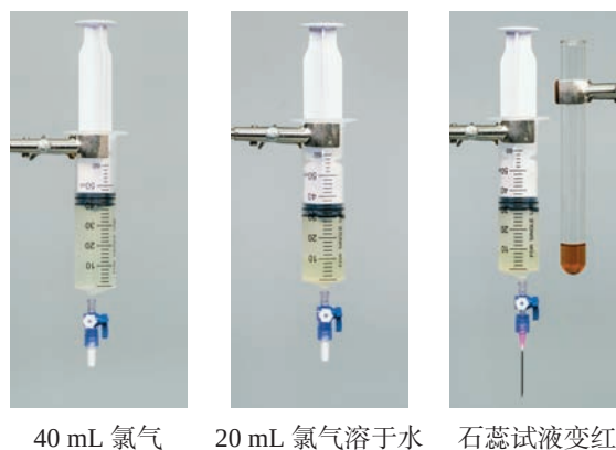
图 2.8 氯气的溶解性及氯水的酸性
