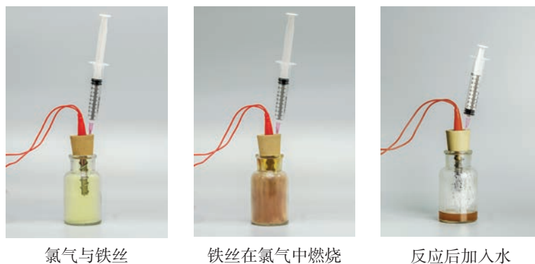
图 2.6 铁丝在氯气中燃烧
