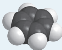
图 7.23 苯分子的空间填充模型
