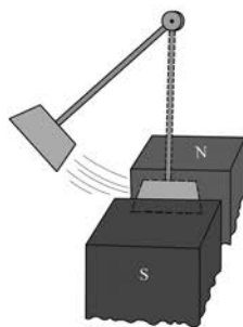
图 7-6 电磁阻尼现象
