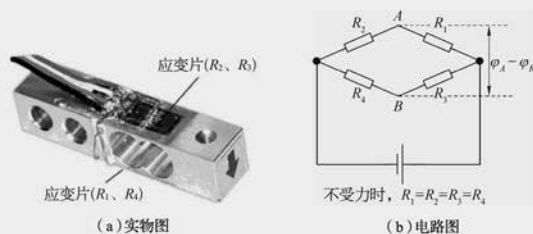
图 9-14 悬臂梁与桥式电路图
