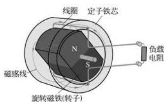
图 7-38 旋转磁极式发电机
