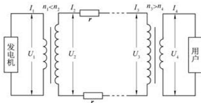
图 7-32 远距离输电原理
