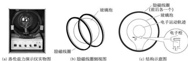
图 5-29 洛伦兹力演示仪
