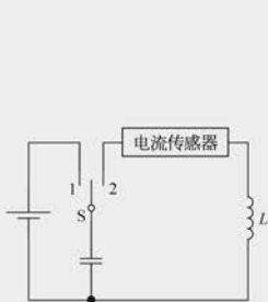
图 8-6 实验电路图
