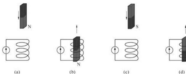
图 6-4 研究感应电流方向的实验过程
