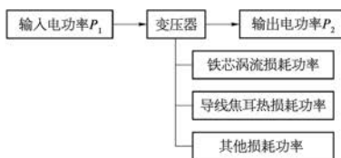
图 7-30 实际变压器的功率转换关系
