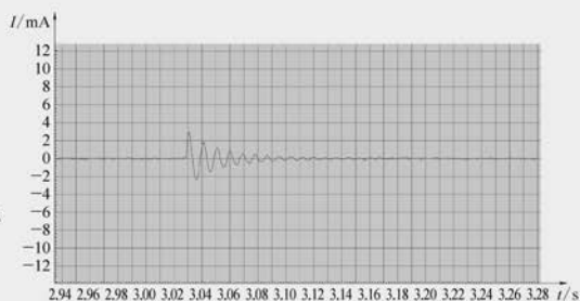
图 8-7 实验记录图
