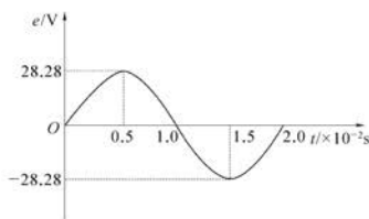
图 7-21 线圈中感应电动势随时间变化的图像
