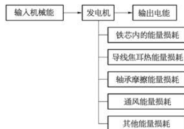
图 7-39 发电机的能量转换关系
