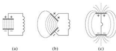
图 8-9 LC 电路的演变过程
