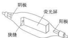
图 5-20 阴极射线管结构
