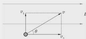
图 6-22 分解导体棒运动速度计算感应电动势
