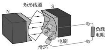
图 7-37 旋转电枢式发电机
