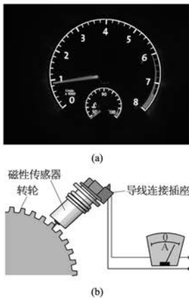
图 6-15 汽车发动机转速表和转速测试装置
