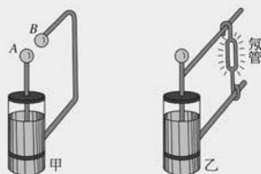
图 8-16 电谐振实验
