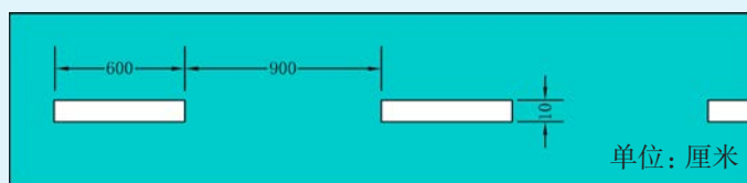
图 3-2-9 高速公路上的车行道分界线示意图
