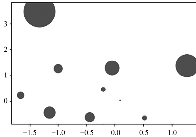
图 4.21 气泡图
