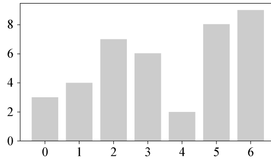
图 4.15 柱形图
