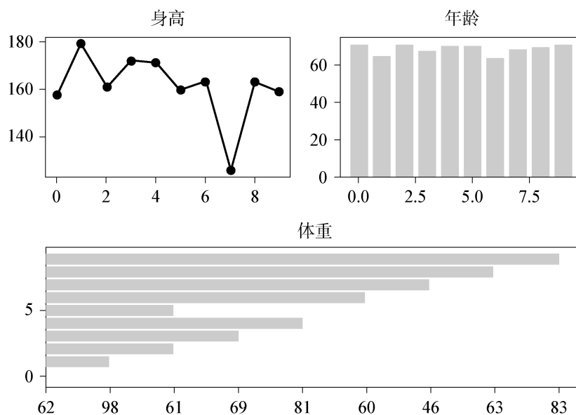
图 4.19 多子图
