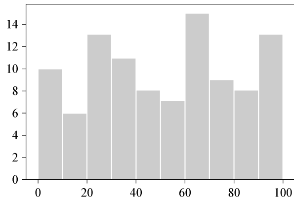
图 4.18 直方图
