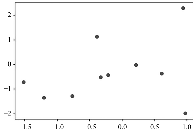
图 4.20 散点图
