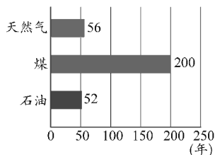
已探明的化石燃料消耗年限图 (2017 年)
