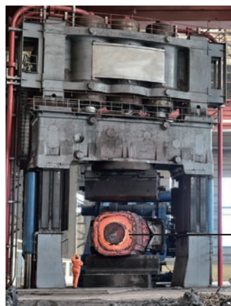
图 3-3-3 钢锭在油压机的压力下变形
