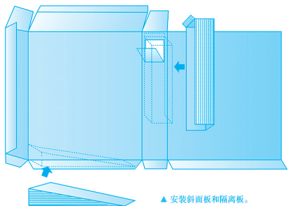
▲ 安装斜面板和隔离板。
