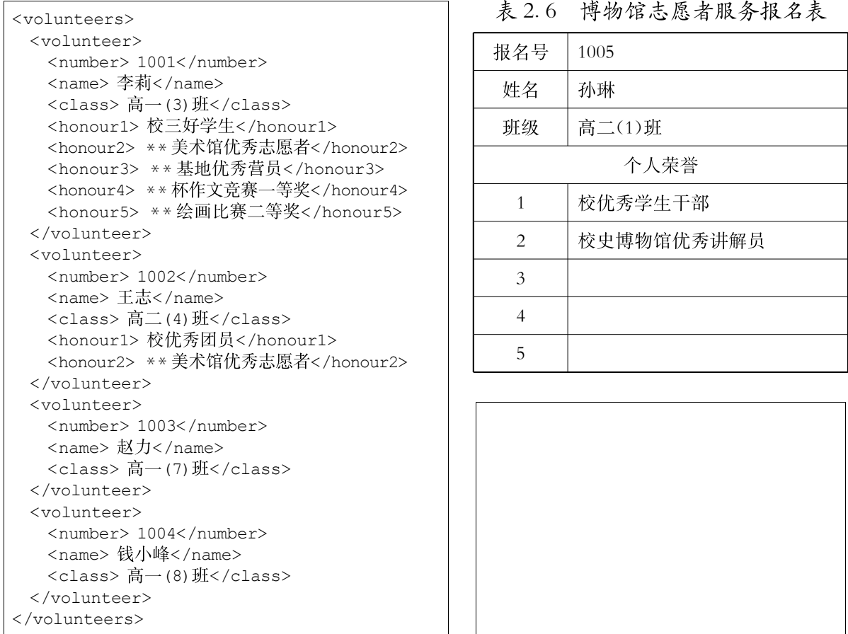
图 2.3 使用 XML 格式存储志愿者报名信息
