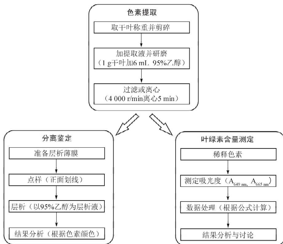
图 4-9 实验流程图
