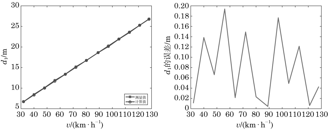
(a) 反应距离 d_1
