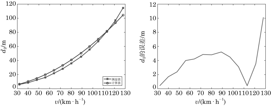
(b) 制动距离 d_2
