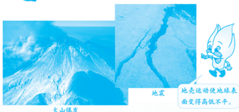
火山爆发
