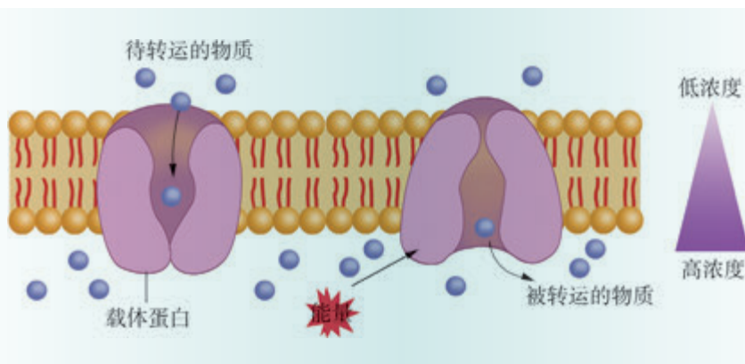
图 4-5 主动运输示意图
