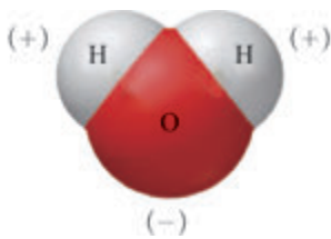
图 2-21 水分子模式图 (显示极性)
