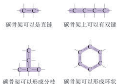
图 2-2 碳骨架示意图
