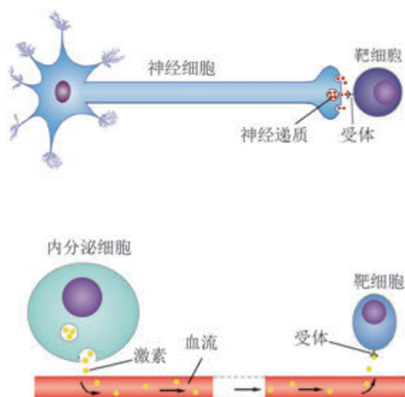
图 3-3 细胞间信号分子传递示意图
