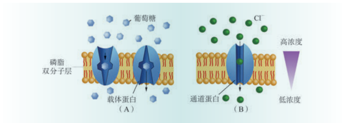
图 4-4 协助扩散示意图
