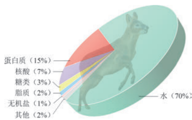
图 2-1 陆生动物体化合物组成的大致比例示意图
