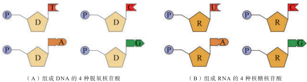
图 2-12 组成 DNA 和 RNA 的核苷酸结构示意图
