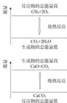
图 5.21 化学反应中的能量变化示意图
