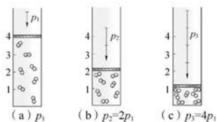
图 6.5 压强对气体浓度影响示意图
