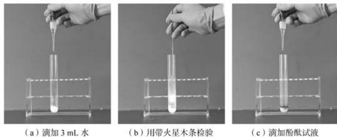
图 5.11 过氧化钠与水反应
