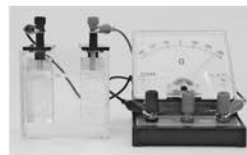
图 5.22 原电池实验装置
