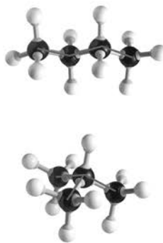
图7.9 正丁烷和异丁烷的球棍模型
