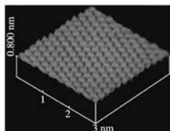
图 10-2 硅片表面原子排列图像
