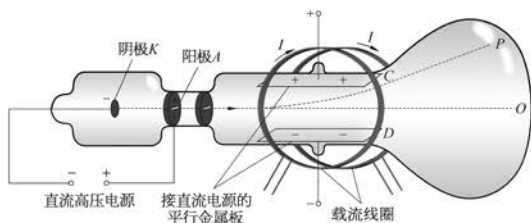
图 13-4 用静电偏转管测电子的比荷
