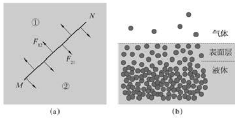
图 11-31 液体的表面张力
