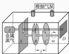
图 10-17 密勒和库士的实验装置示意图
