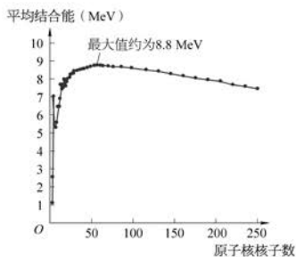
图 15-14 平均结合能与核子数的关系
