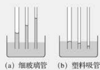
图 11-34 水对玻璃浸润、对塑料不浸润
