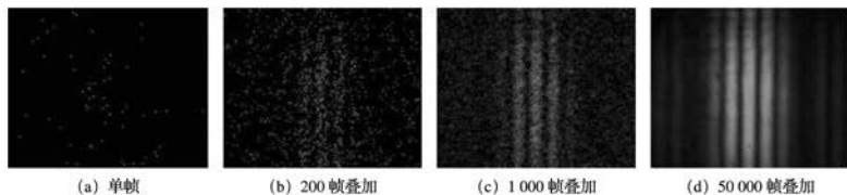
图 14-13 光子逐个通过双缝后的干涉图样
