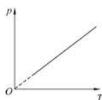
图 11-22 等容线
