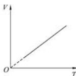
图 11-23 等压线
