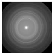
(b) 电子经多晶体衍射的图样
