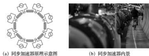
图 15-30 同步加速器
