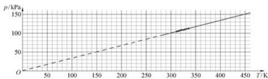
图 11-21 气体压强 p 与热力学温度 T 的关系
