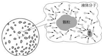
图 10-11 颗粒受到液体分子的撞击
