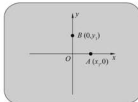
图 11-46
