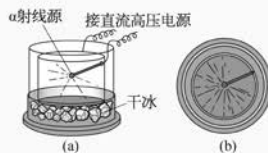
图15-9 云室
