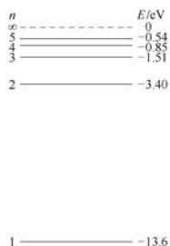
图 13-15 氢原子的能级图
