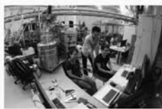
图 15-33 上海同步辐射光源内的线站
