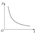
图 11-12 等温线
