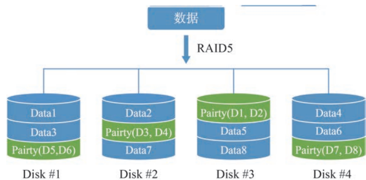
图 3.7 某磁盘阵列
