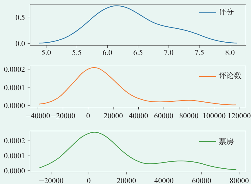
图 5.4 概率密度函数图
