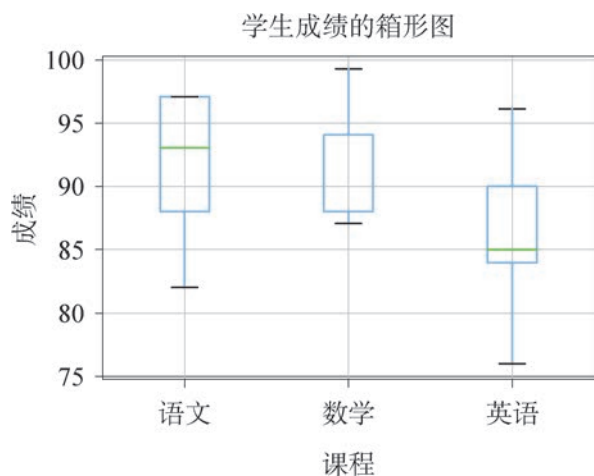
图 4.9 5 位学生成绩的箱形图
