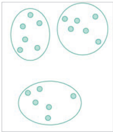
聚类后的数据分布
