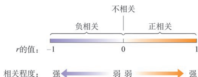
图 4.16 解读相关系数 r
