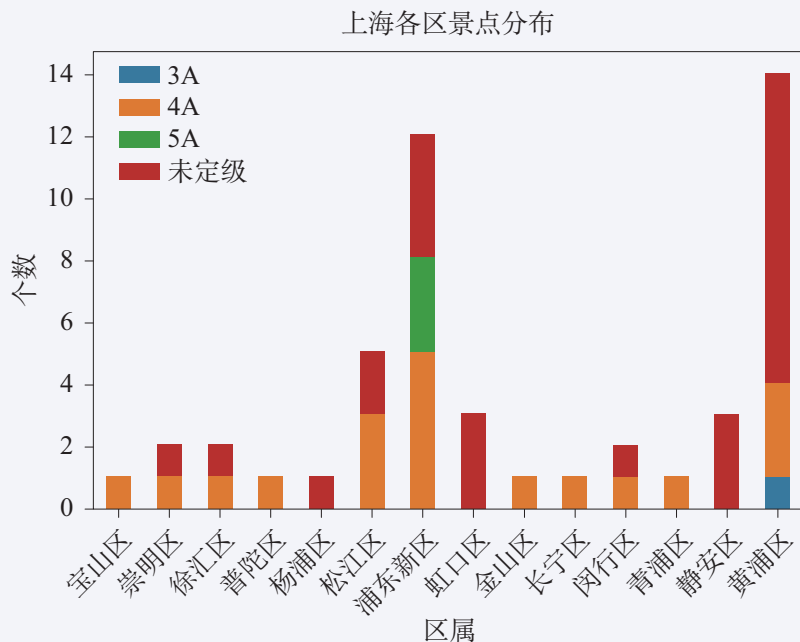
图 4.15 上海各区景点分布的堆积柱形图
