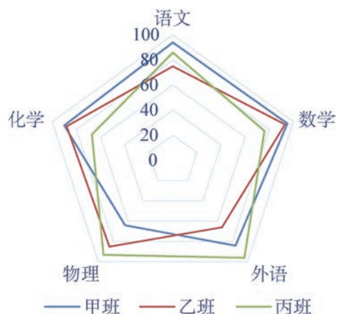
图 4.10 某学校 3 个班 5 门课程平均成绩雷达图
