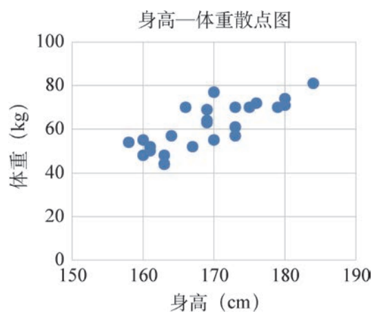
图 4.8 身高—体重散点图
