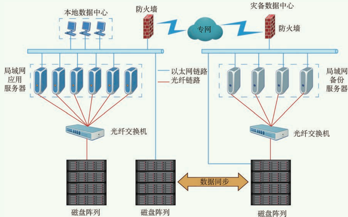
图 3.10 数据备份系统
