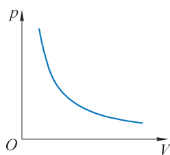
图 11-12 等温线
