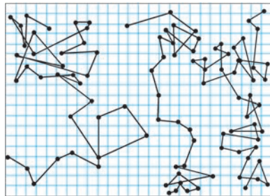
图 10-10 布朗运动
