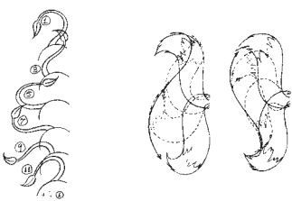
曲线运动：两个弹跳运动的相向运动
