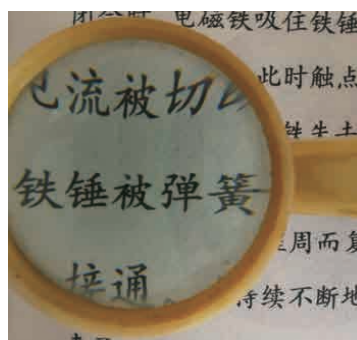
用凸透镜看到的像
