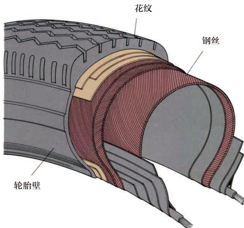
轮胎结构
