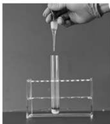
(c) 滴加酚酞试液
