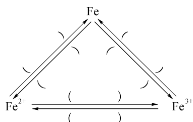
图 5 不同价态铁元素之间的转化
