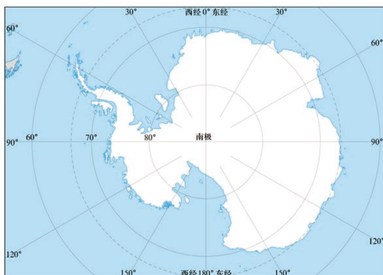
图 9 南极地区
