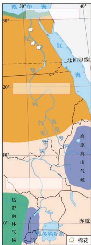
图 14 尼罗河流域
