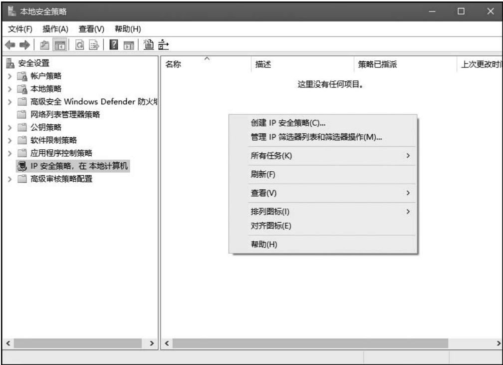
图 4-8 单击“创建 IP 安全策略”
