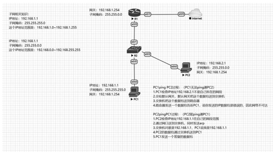
图5-9 网络拓扑图
