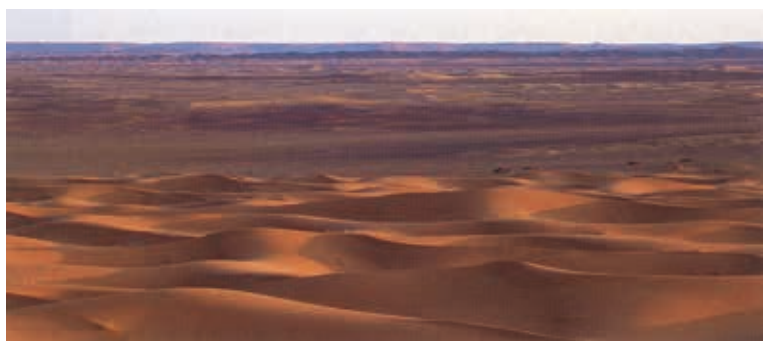
撒哈拉沙漠的一部分：这里几乎不下雨
