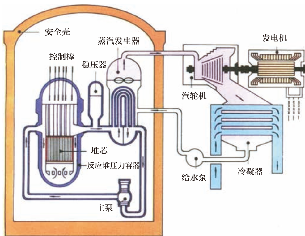
核蒸汽供应系统
