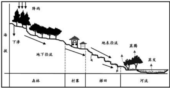
元阳梯田生态系统示意图
