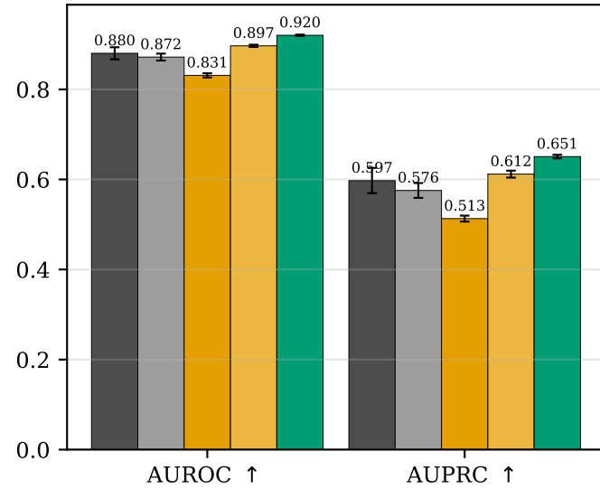
Aionoscope (AUROC/AUPRC)
